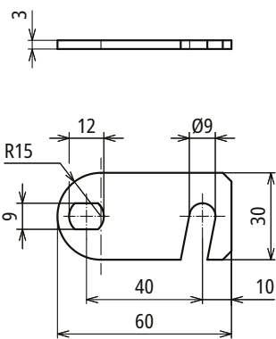
Maßbild
