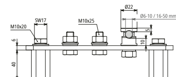
Maßbild
