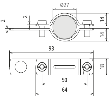
Maßbild
