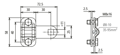
Maßbild
