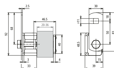
Maßbild
