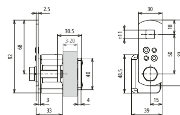
Maßbild
