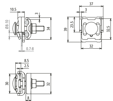
Maßbild
