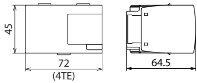
Maßbild
