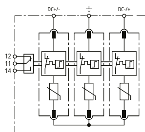
Prinzipschaltbild
