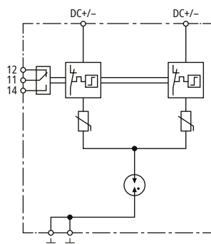
Prinzipschaltbild
