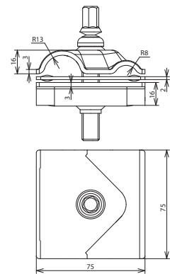
Maßbild
