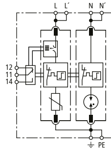
Prinzipschaltbild
