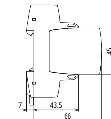
Maßbild
