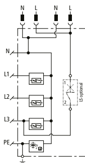
Prinzipschaltbild
