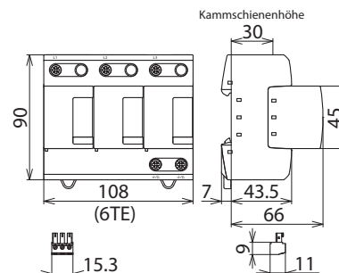
Maßbild
