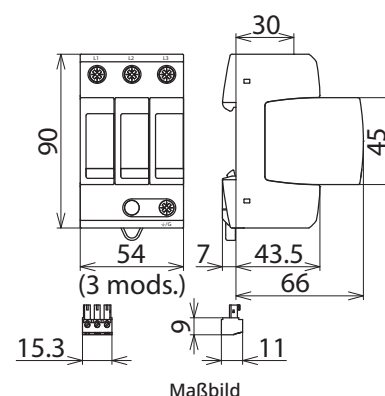
Maßbild
