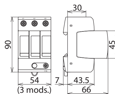
Maßbild
