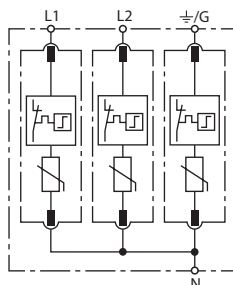
Prinzipschaltbild
