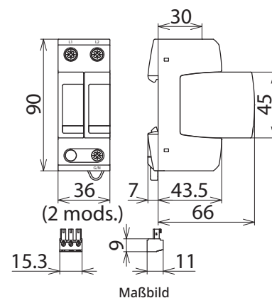
Maßbild
