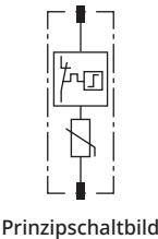
Prinzipschaltbild
