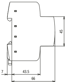
Maßbild
