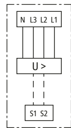
Prinzipschaltbild
