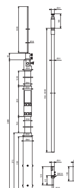
Maßbild
