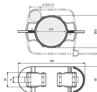
Maßbild
