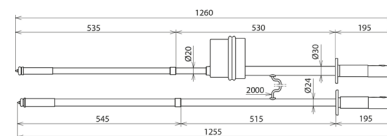
Maßbild
