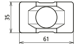
Maßbild
