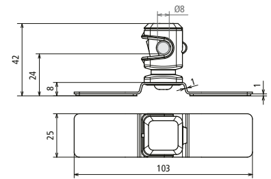
Maßbild
