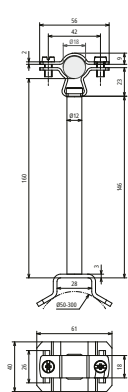
Maßbild
