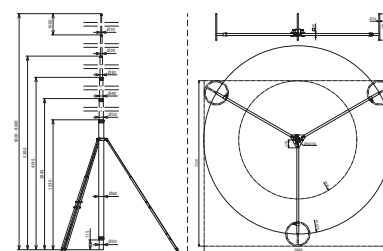
Maßbild
