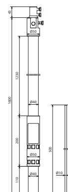
Maßbild
