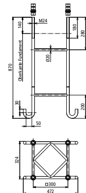
Maßbild
