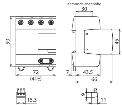
Maßbild
