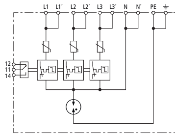
Prinzipschaltbild
