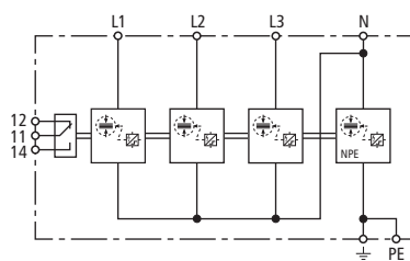
Prinzipschaltbild
