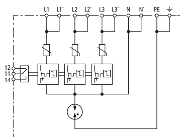
Prinzipschaltbild
