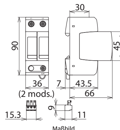
Maßbild
