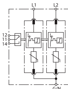
Prinzipschaltbild
