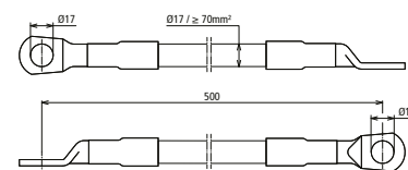
Maßbild
