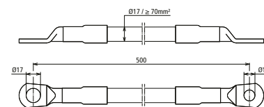
Maßbild
