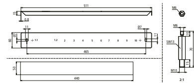
Maßbild
