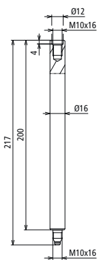
Maßbild
