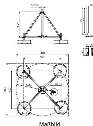
Maßbild
