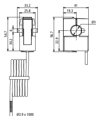
Maßbild
