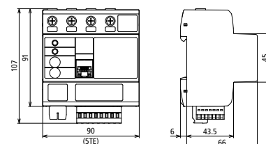
Maßbild
