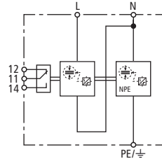
Prinzipschaltbild
