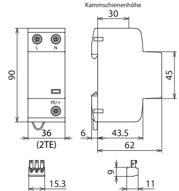
Maßbild
