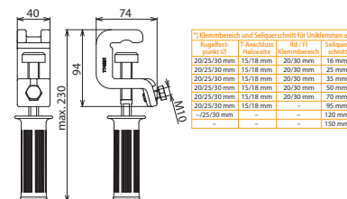
Maßbild
