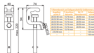
Maßbild
