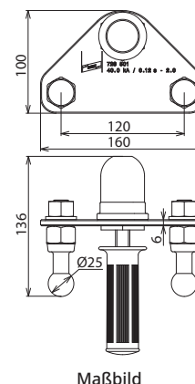
Maßbild
