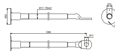
Maßbild
