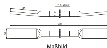
Maßbild
