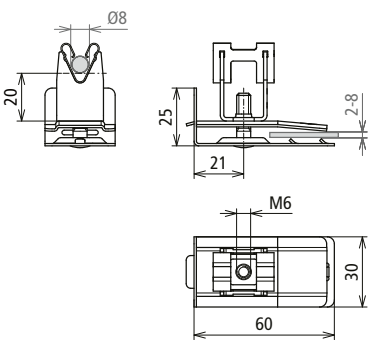
Maßbild
