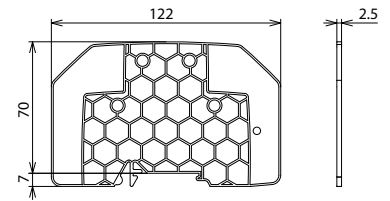
Maßbild
